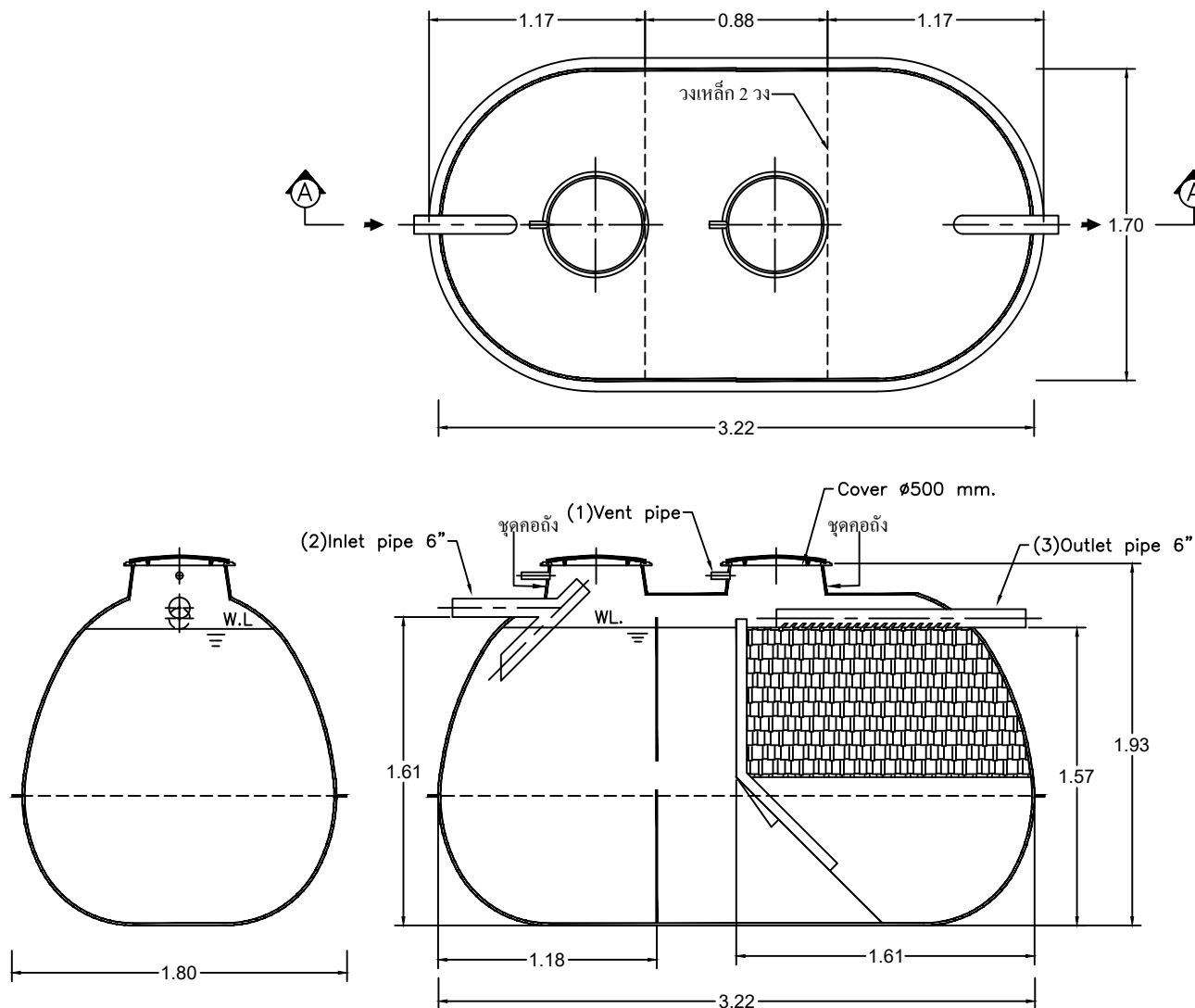
SECTION A-A
