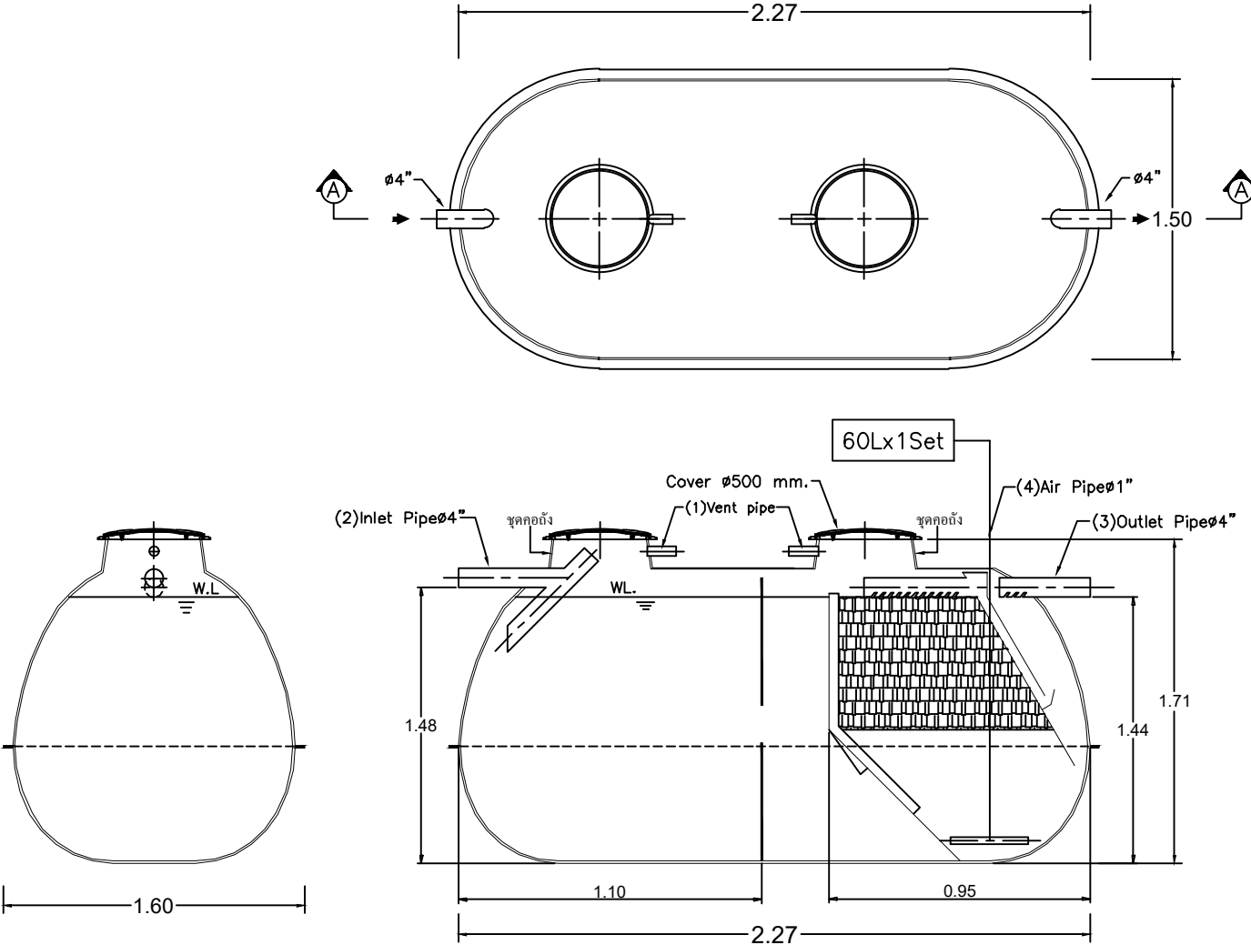
SECTION A-A
