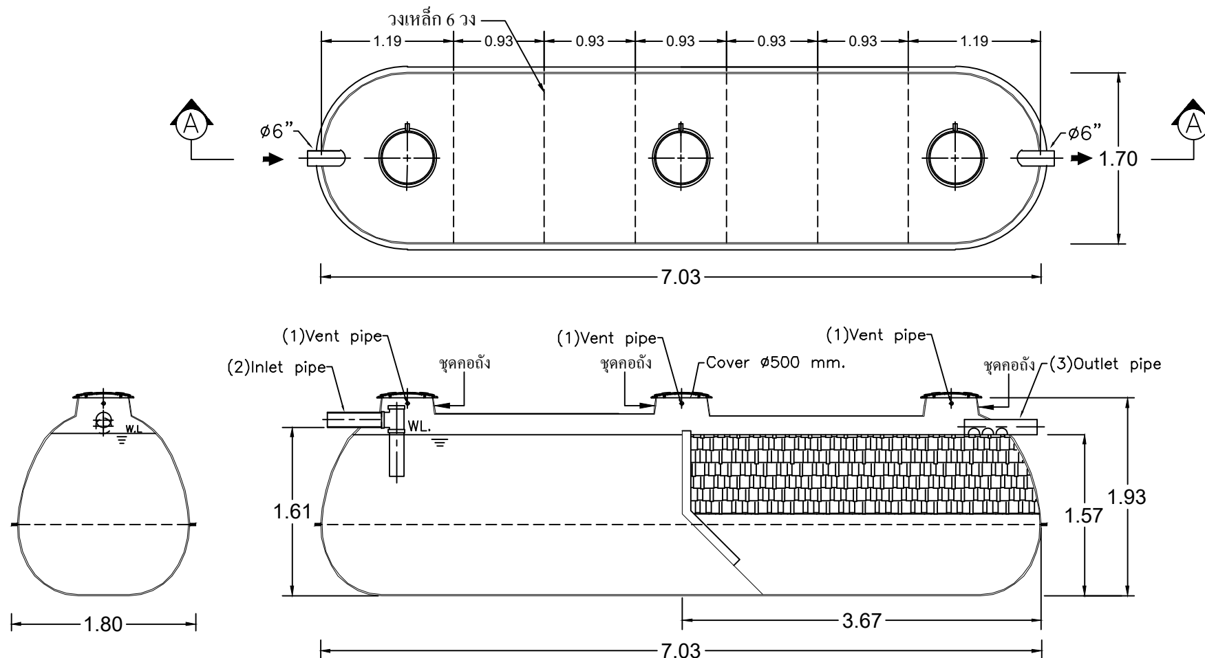
SECTION A-A
