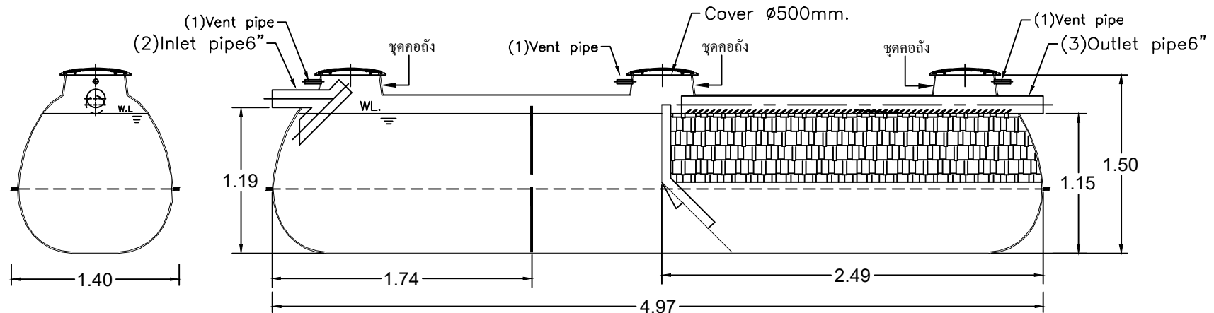
SECTION A-A
