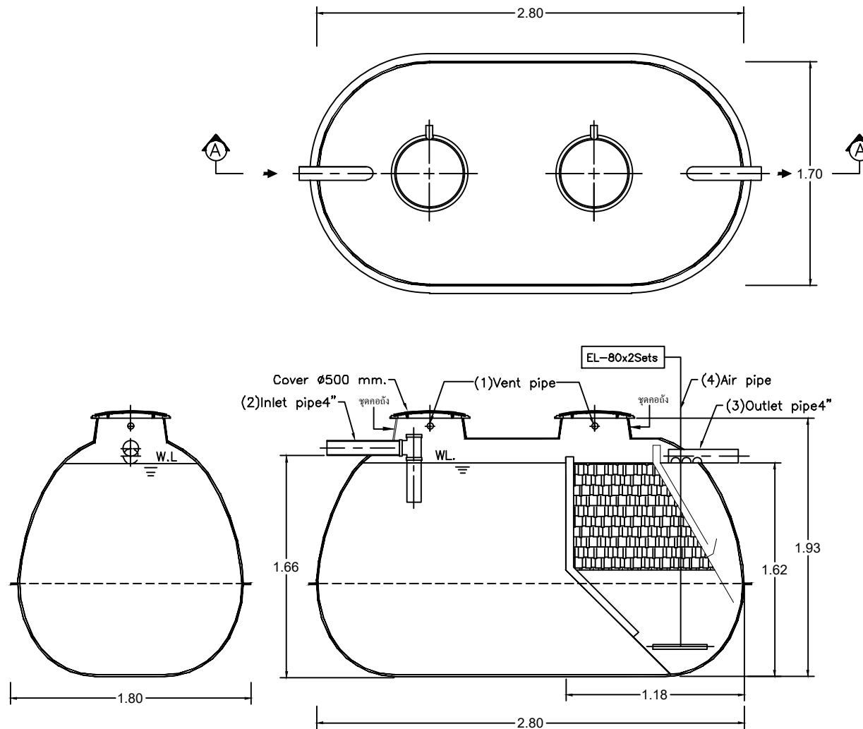
SECTION A-A
