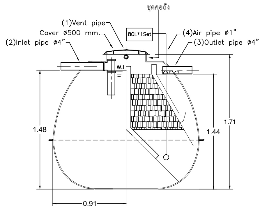
SECTION A-A
