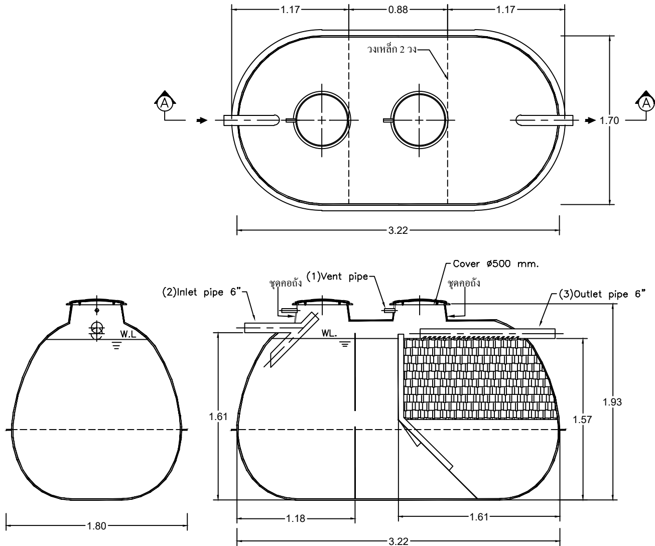
SECTION A-A
