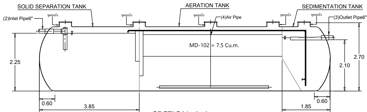
SECTION A-A
