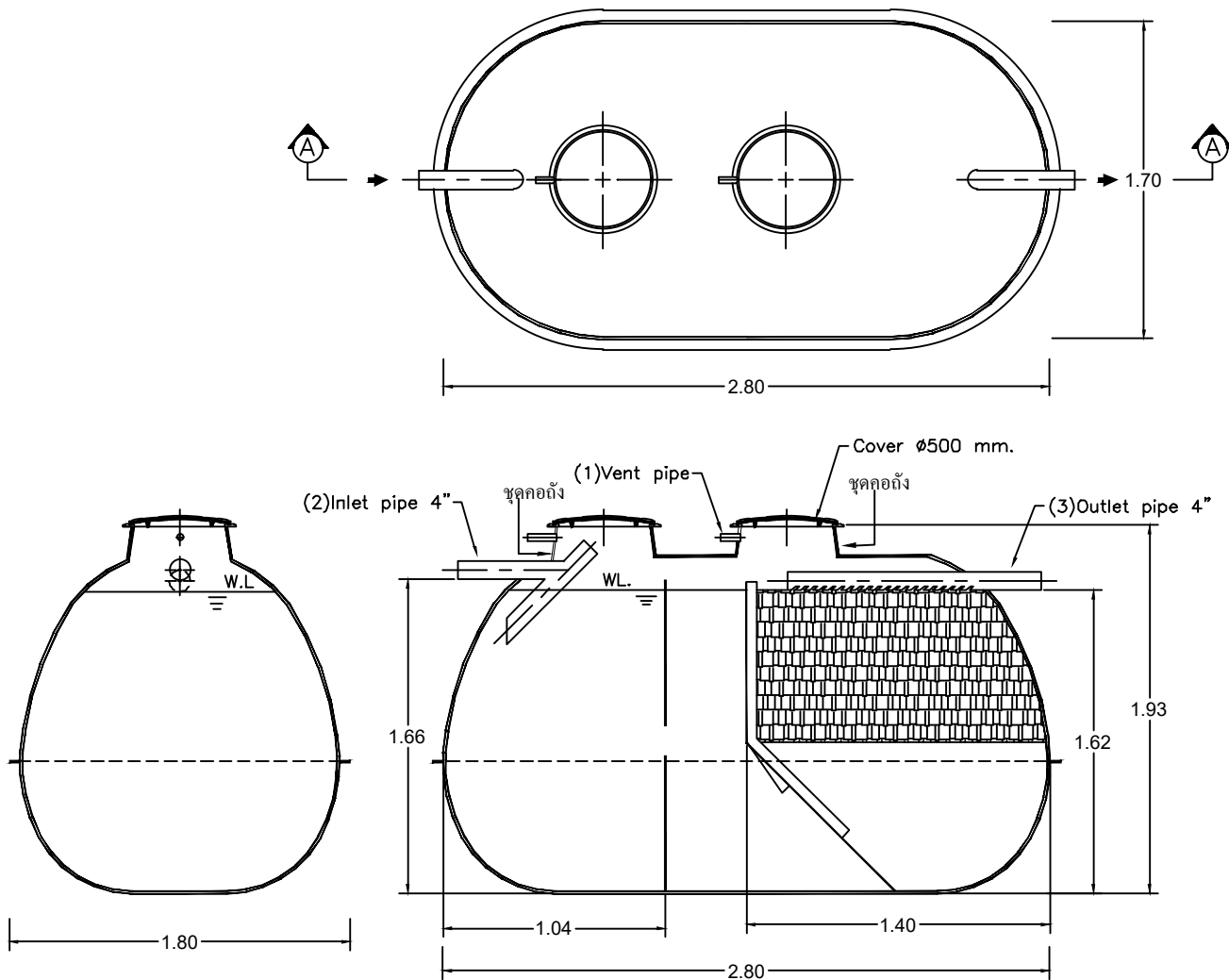
SECTION A-A
