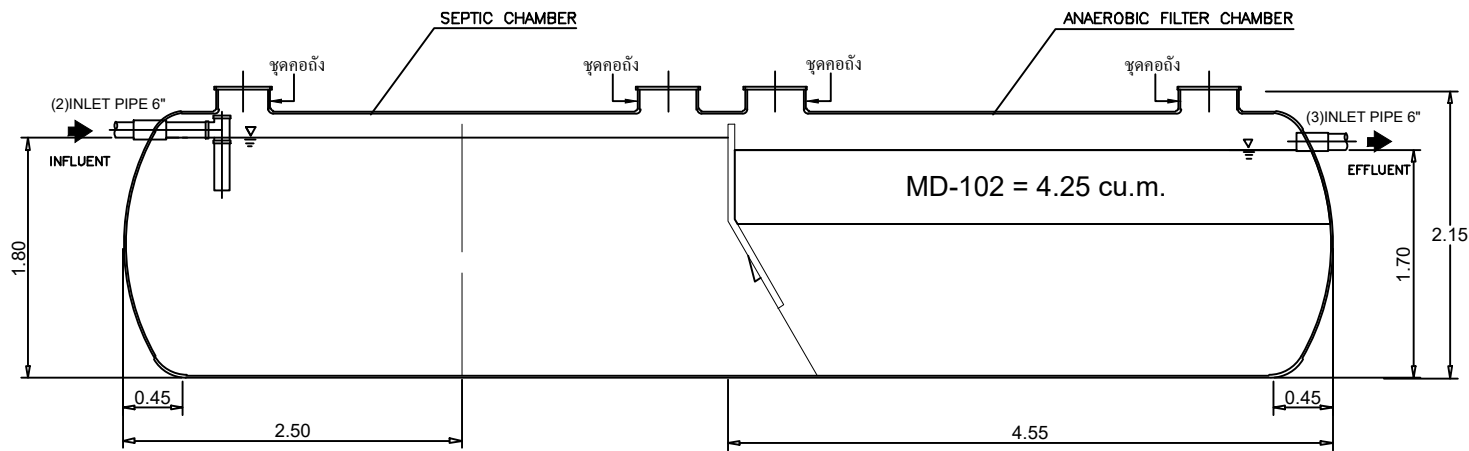
SECTION A-A
