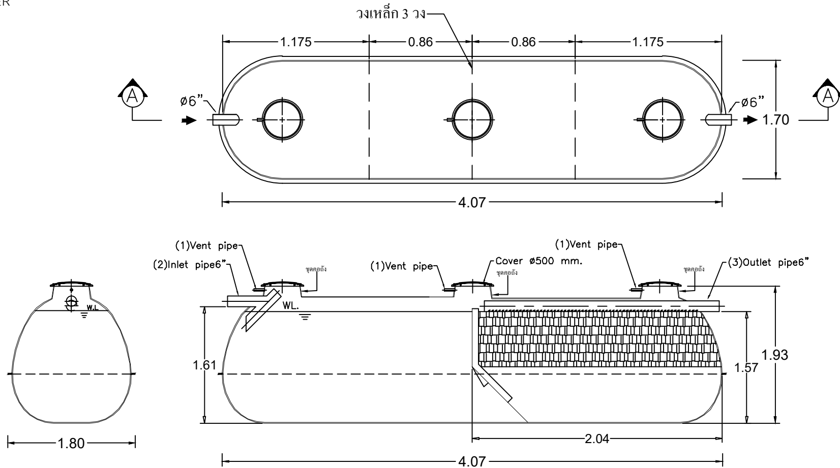
SECTION A-A
