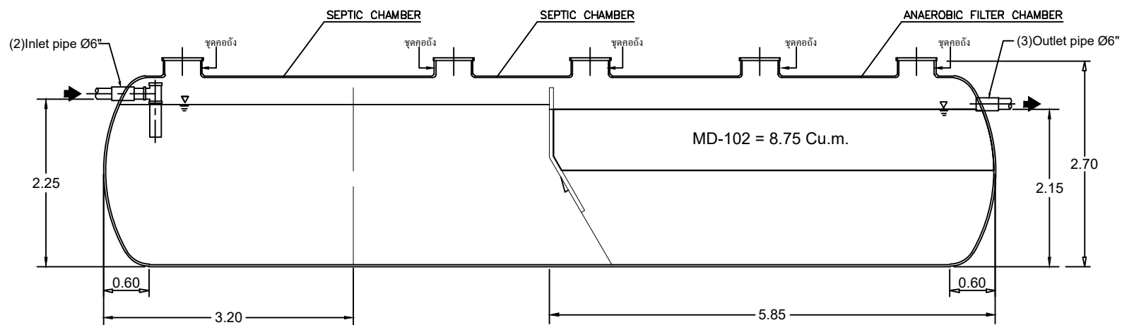
SECTION A-A
