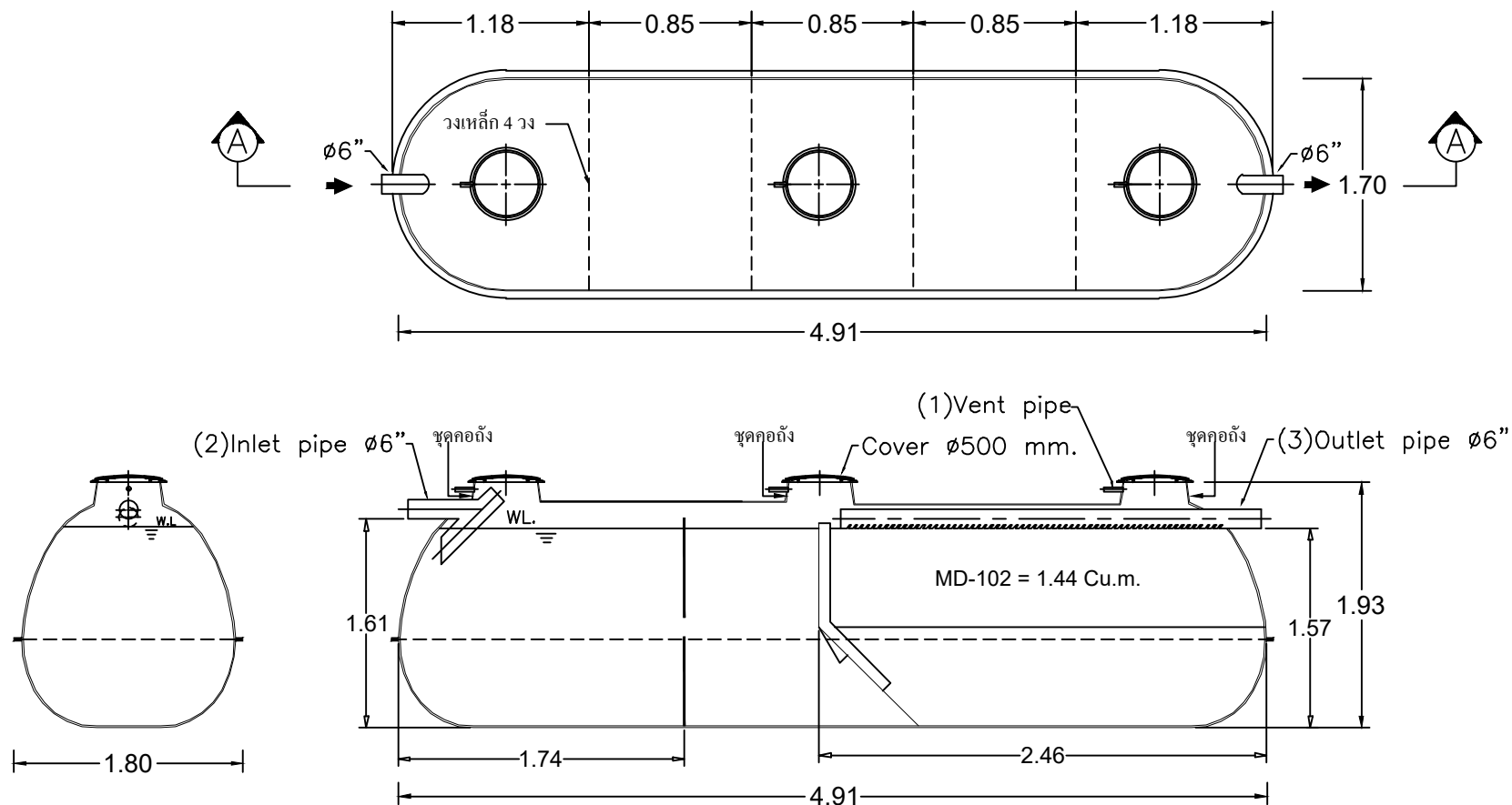
SECTION A-A
