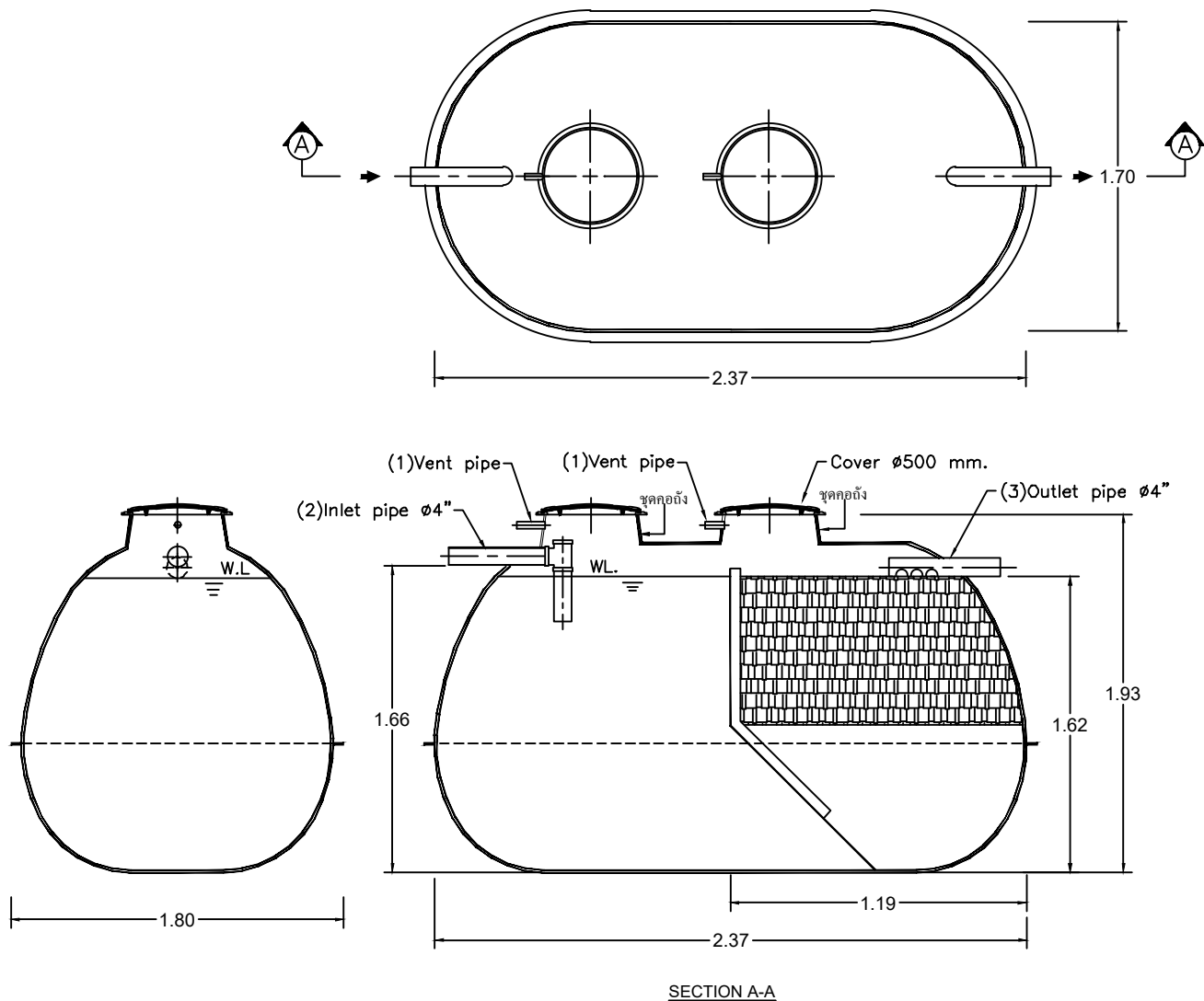
SECTION A-A
