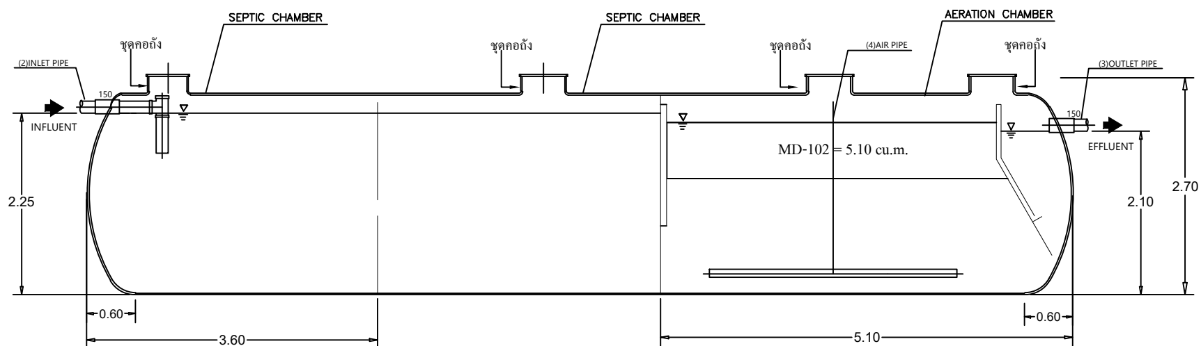
SECTION A-A
