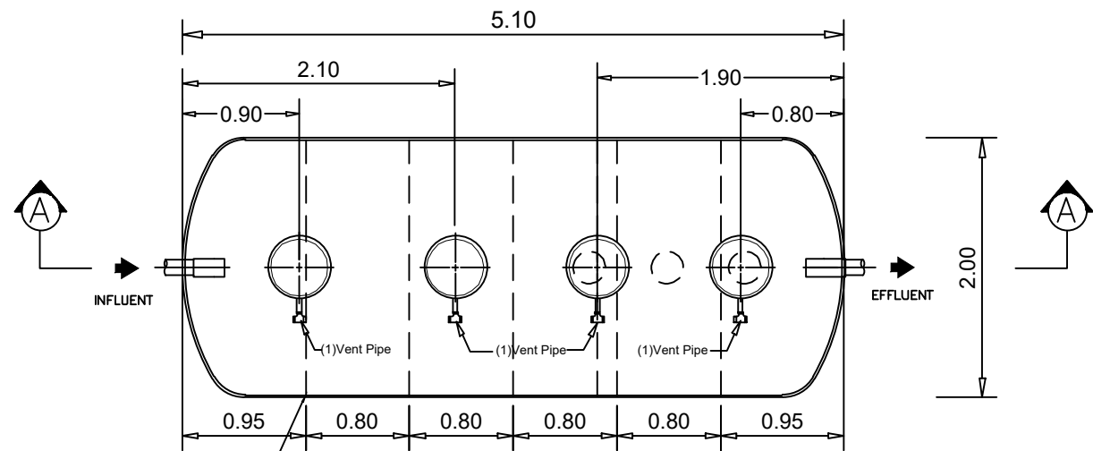
วงเหล็ก 5 วง STAR TANK MODEL SSA-2013Z
