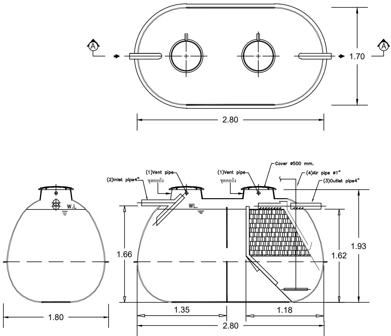
SECTION A-A
