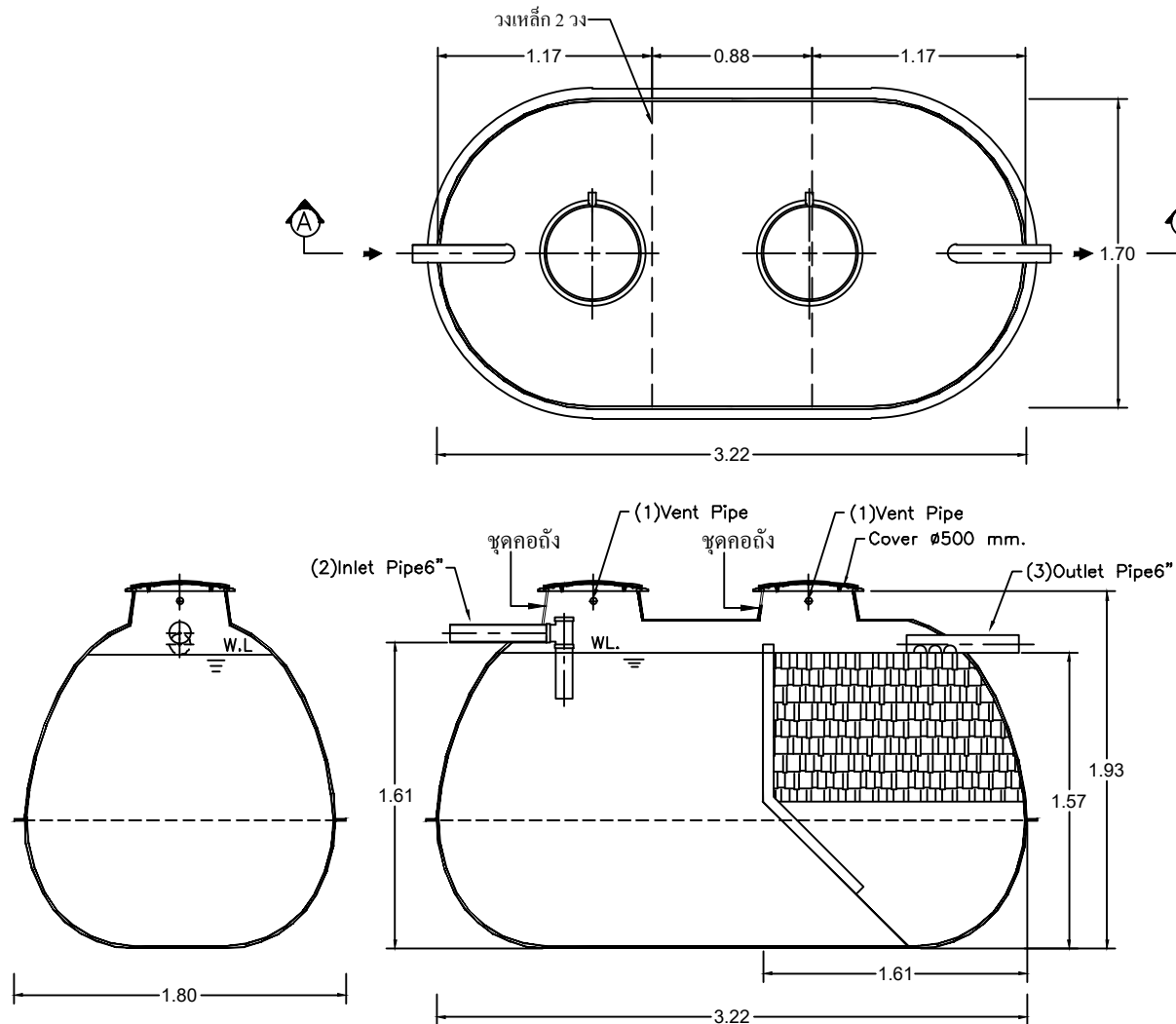
SECTION A-A
