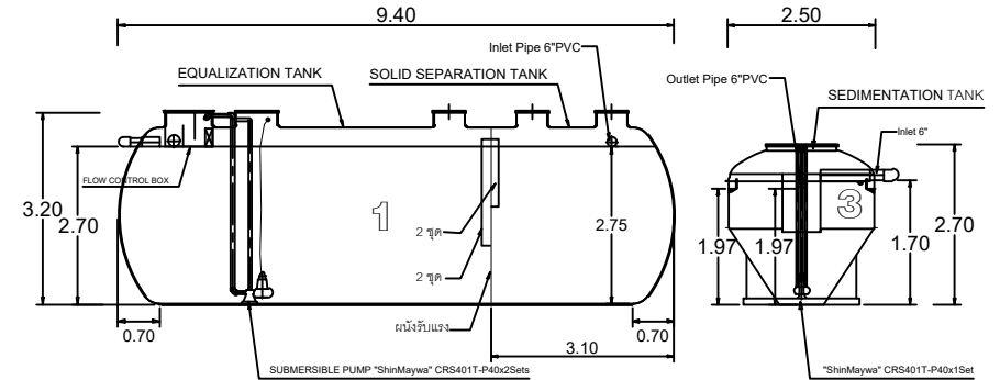
SECTION A-A
