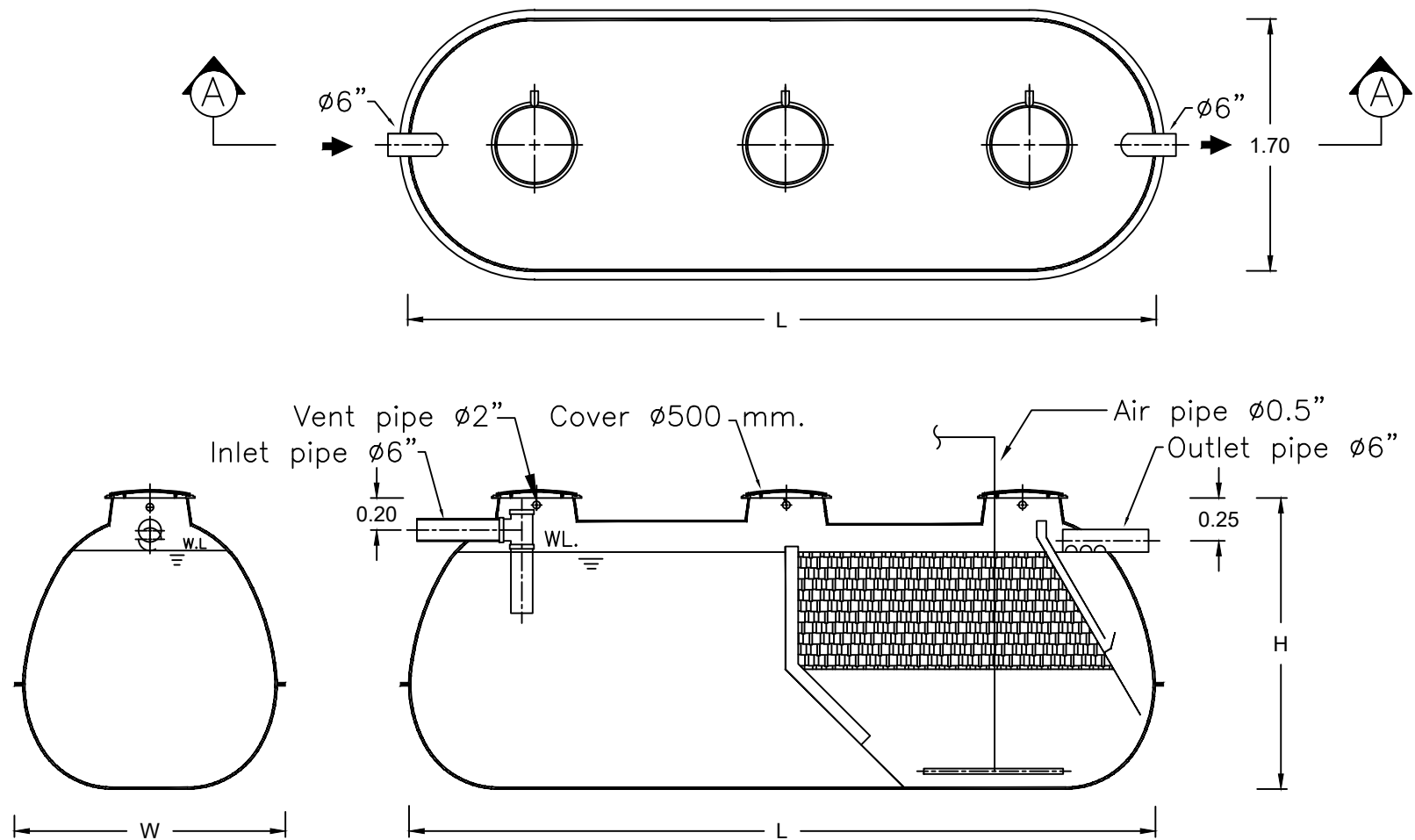
SECTION A-A
