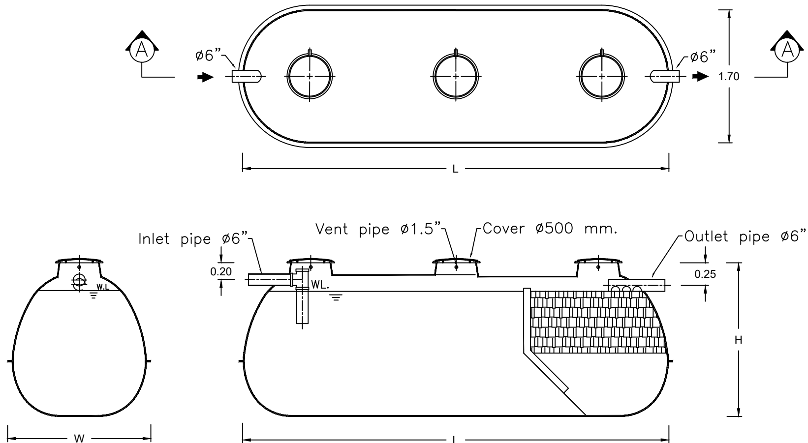
SECTION A-A
