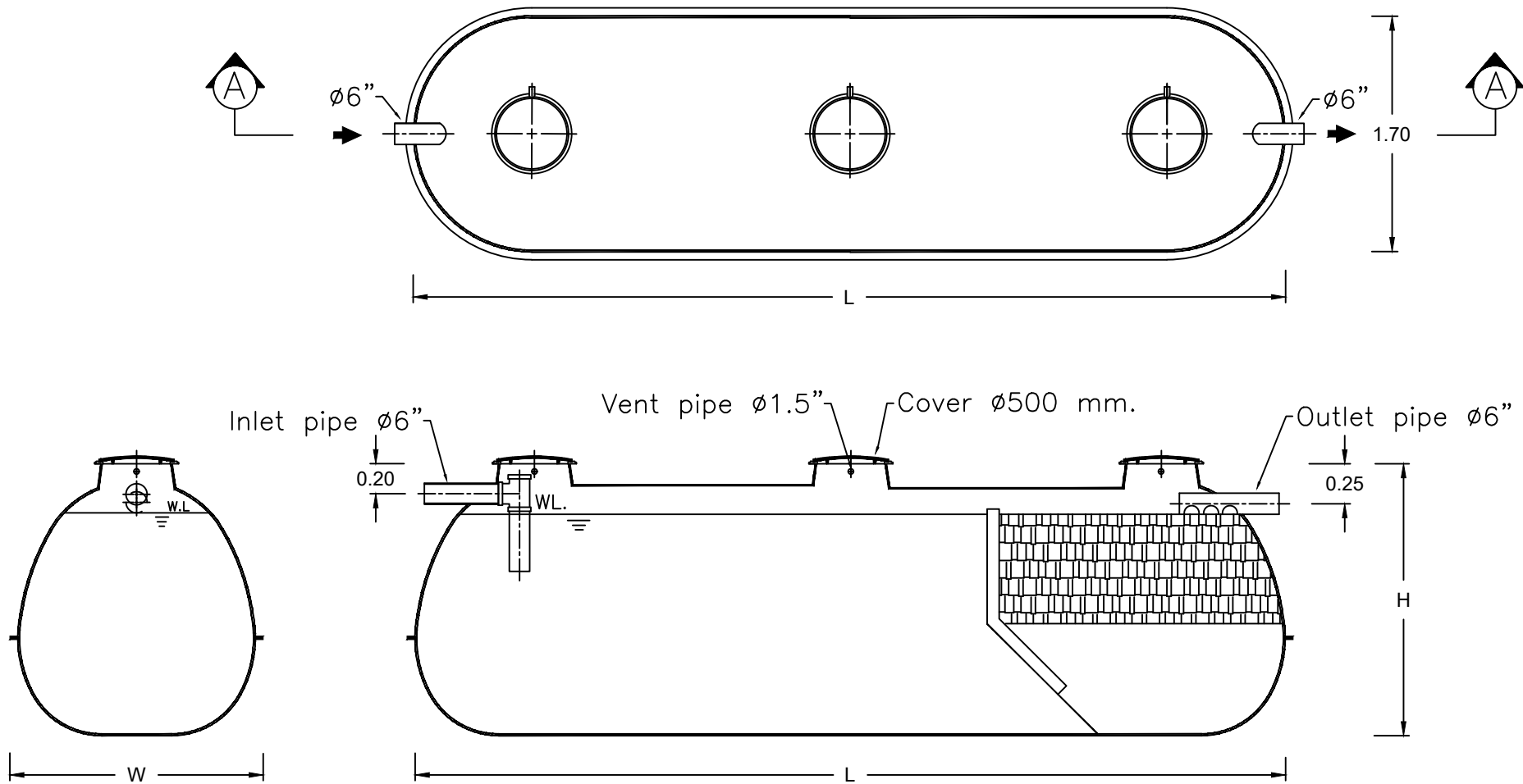
SECTION A-A
