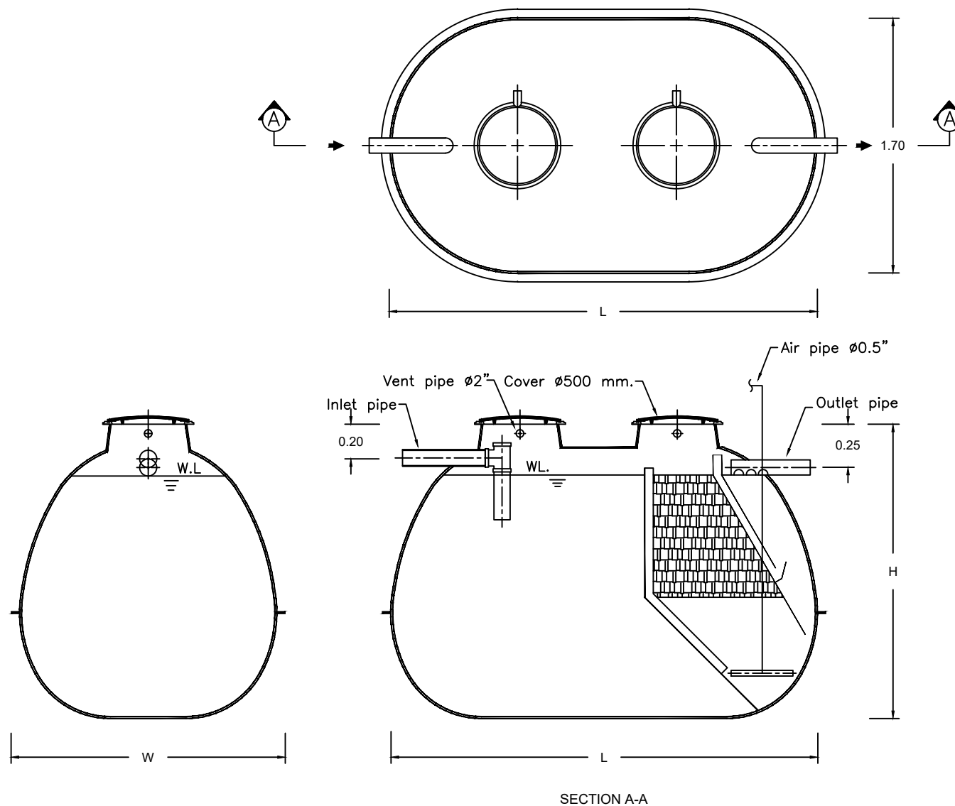
SECTION A-A
