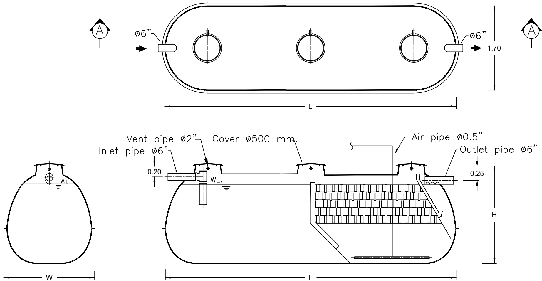
SECTION A-A
