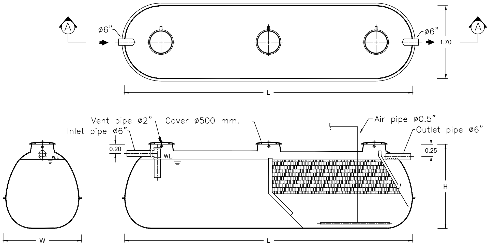
SECTION A-A
