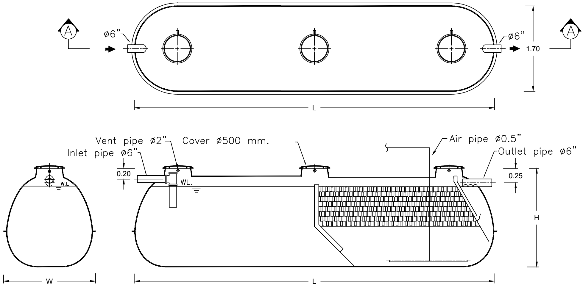
SECTION A-A
