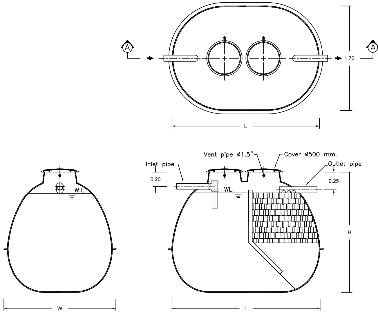
SECTION A-A
